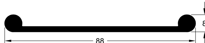
CIA 6194 (EPDM 70 Shore A)
