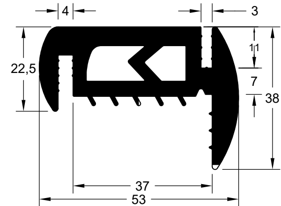
CIA 9152 (EPDM 63 Shore A)
