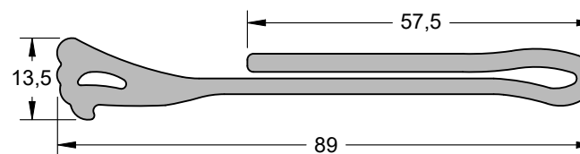
CIA 4272 (EPDM 10 Shore A)
