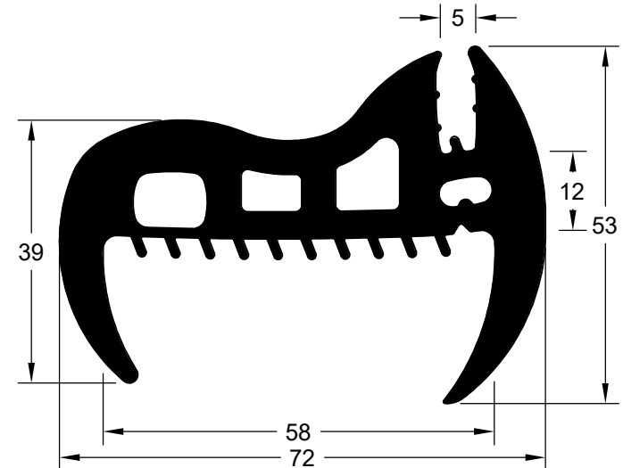
CIA 9123 (EPDM 70 Shore A)
