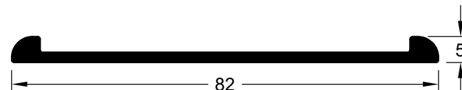
CIA 7052 (TPE 70 Shore A)
