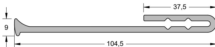
CIA 4283 (EPDM 10 Shore A)
