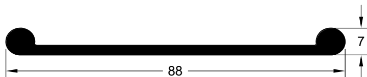
CIA 7051 (TPE 70 Shore A)
