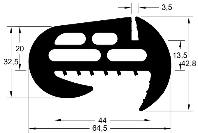
CIA 16022 (EPDM 70 Shore A)
