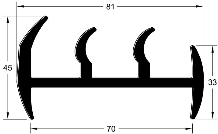
CIA 6162 (EPDM 80 Shore A)
