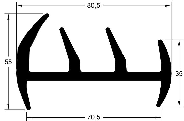
CIA 16857 (EPDM 75 Shore A)
