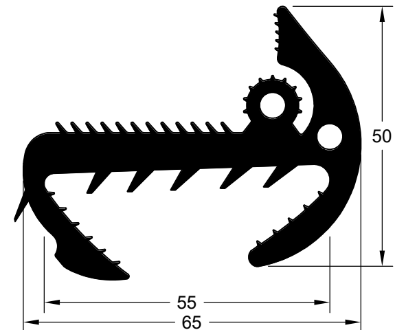
CIA 9159 (EPDM 70 Shore A)
