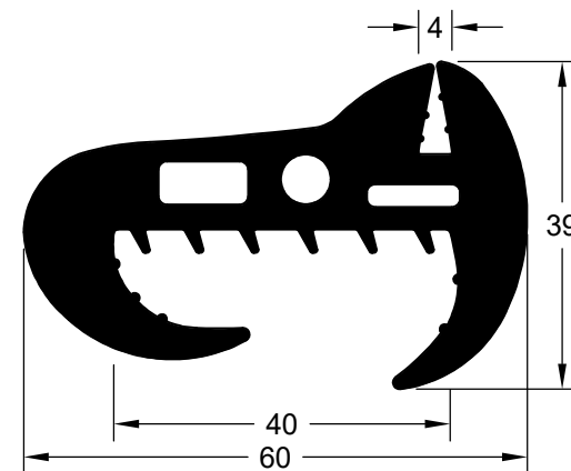
CIA 9083 (EPDM 63 Shore A)
