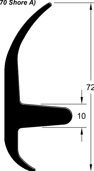
CIA 15073 (EPDM 70 Shore A)
