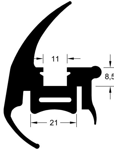
CIA 9154 (EPDM 70 Shore A)
