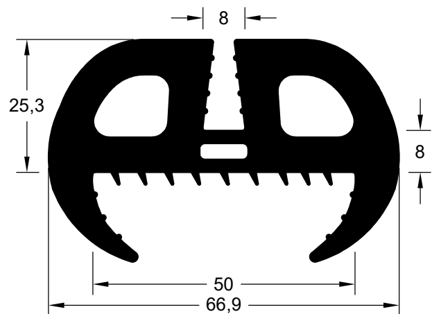
CIA 17263 (EPDM 63 Shore A)
