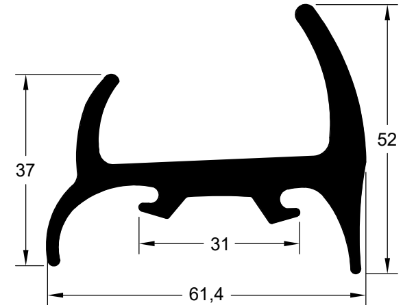
CIA 6339 (EPDM 80 Shore A)
