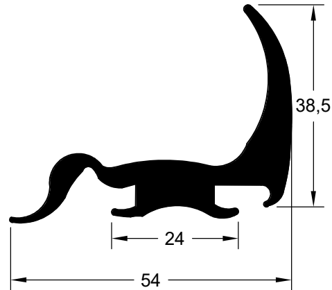
CIA 6340 (EPDM 80 Shore A)
