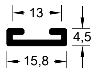
CIA 17518 (EPDM 70 Shore A)
