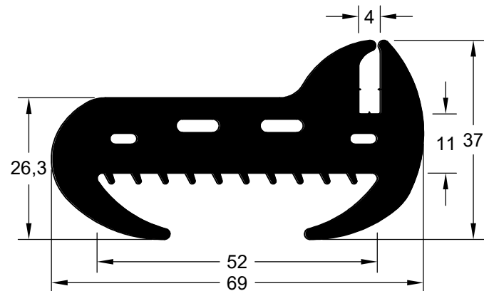
CIA 9145 (EPDM 63 Shore A)
