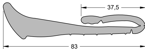
CIA 4166 (EPDM 10 Shore A)
