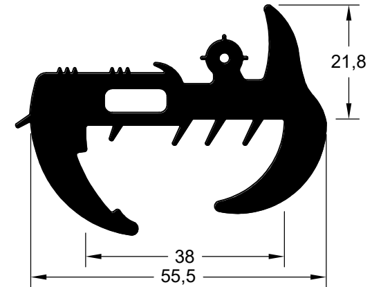
CIA 9159 (EPDM 70 Shore A)
