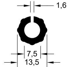
CIA 14383 (EPDM 70 Shore A)
