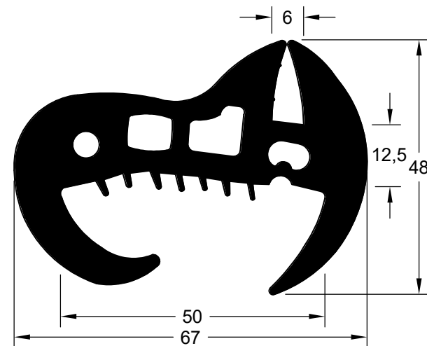
CIA 9140 (EPDM 63 Shore A)
