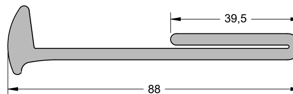
CIA 4272 (EPDM 10 Shore A)
