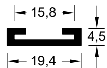
CIA 17517 (EPDM 70 Shore A)
