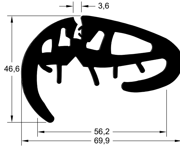
CIA 9092 (EPDM 63 Shore A)
