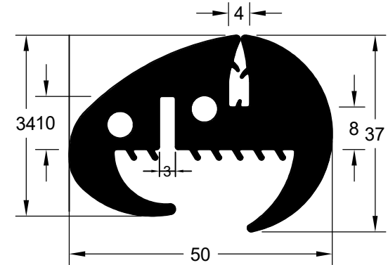
CIA 9126 (EPDM 63 Shore A)
