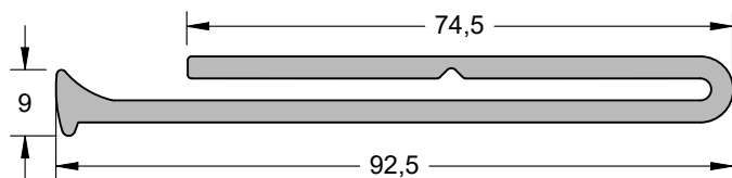
CIA 4284 (EPDM 10 Shore A)
