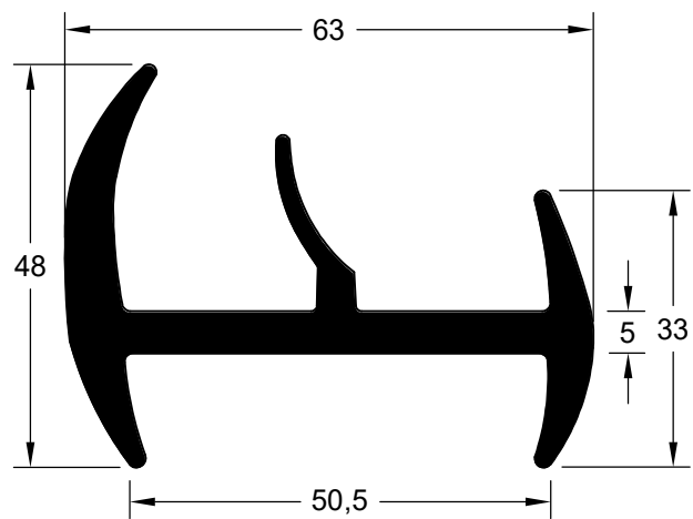
CIA 17521 (EPDM 75 Shore A)
