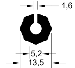
CIA 9162 (EPDM 70 Shore A)
