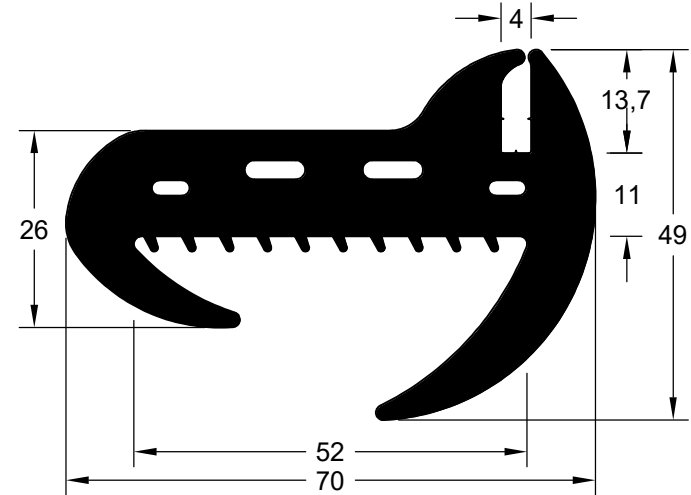
CIA 9129 (EPDM 70 Shore A)
