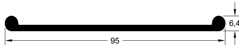
CIA 7050 (TPE 70 Shore A)
