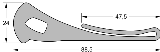
CIA 4178 (EPDM 10 Shore A)
