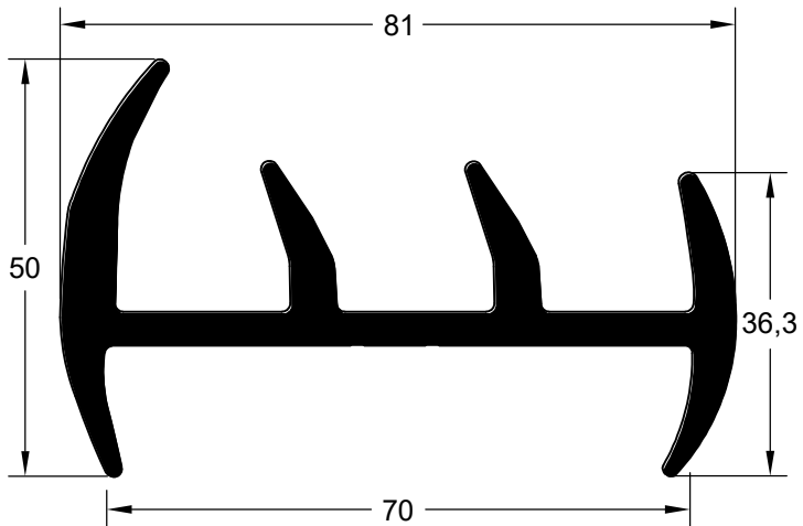
CIA 19879 (EPDM 75 Shore A)
