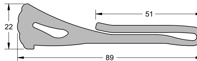
CIA 4274 (EPDM 10 Shore A)
